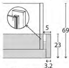
Draufsicht Schrank inkl. PPT-Rahmen
